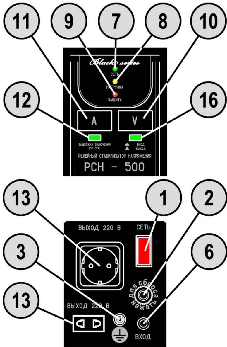
Рис. 1 а). РСН-500/1000/1500/2000
