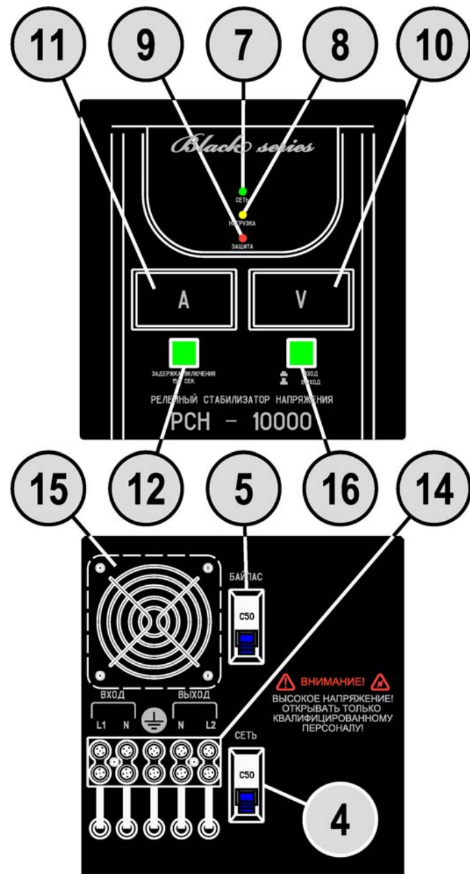
Рис. 1 б). РСН-3000/5000/8000/10000
